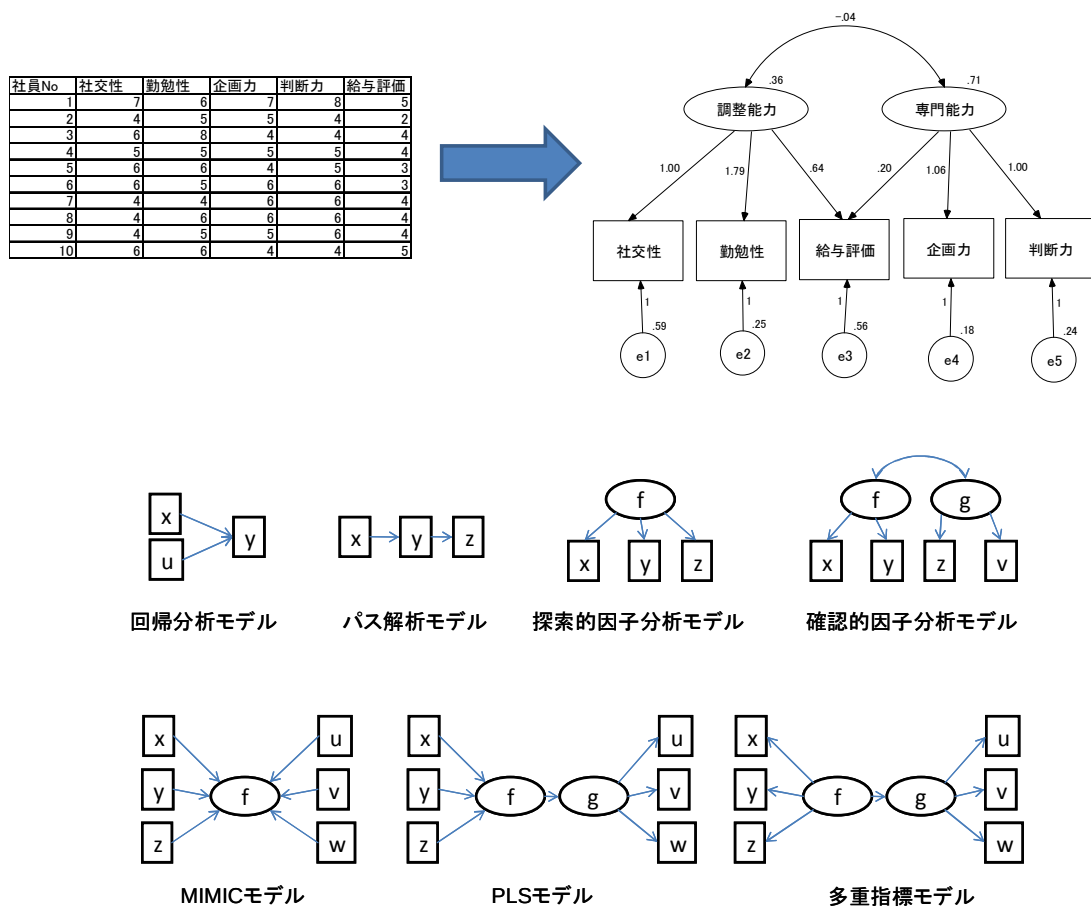
Figure 46 共分散構造分析の概念図
